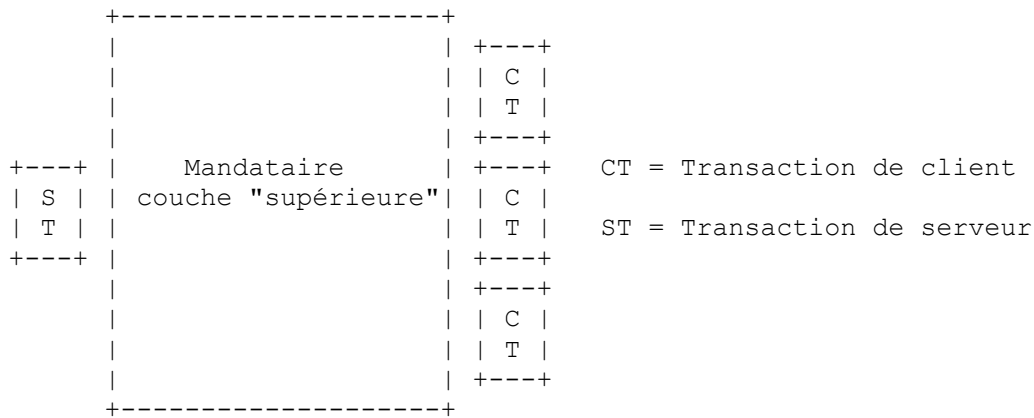
Figure 3 : Modèle de mandataire à états pleins
