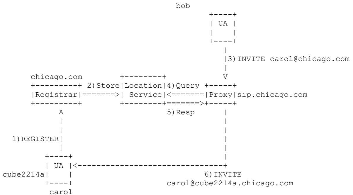
Figure 2 : Exemple de REGISTER
