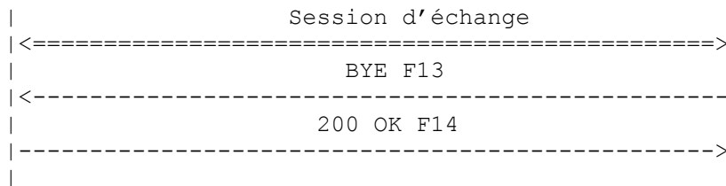
Figure 1 : Exemple d'établissement de session SIP avec le trapézoïde SIP
